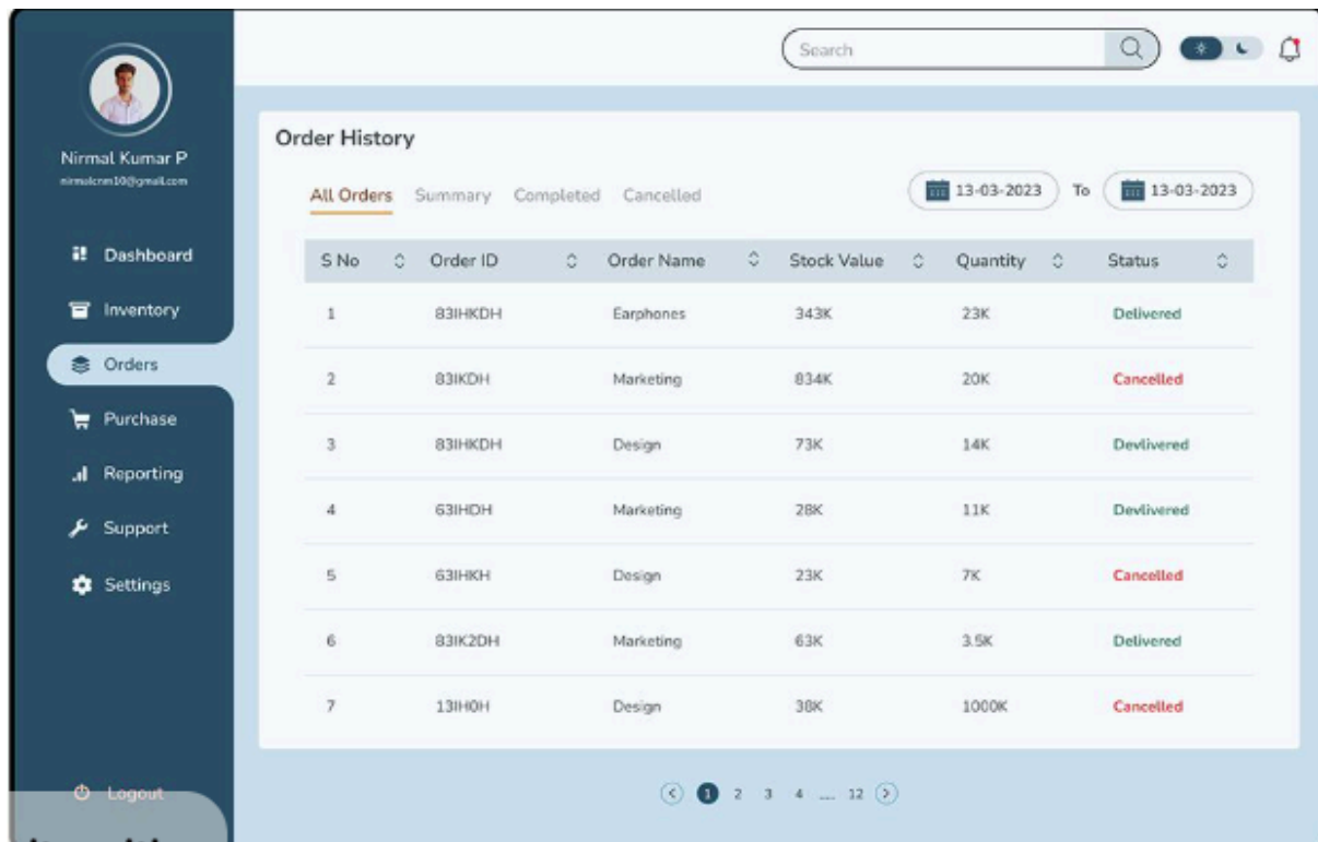
Imagen 1
