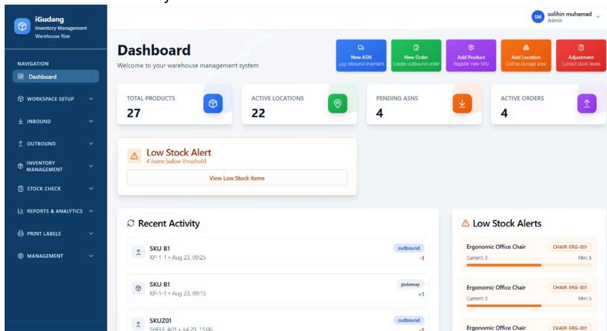
Imagen 2
